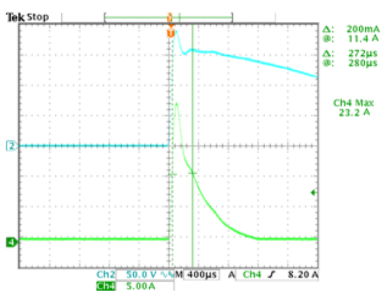
CH2 : AC Input Voltage CH4 : Input current
