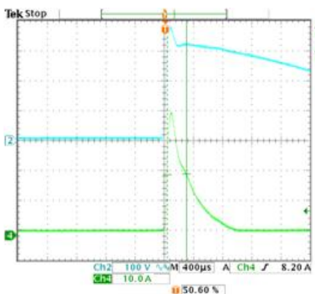
CH2 : AC Input Voltage CH4 : Input current
